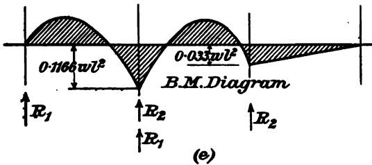
FIG. 65 (d) and (e).—Three spans, one bay unloaded.
